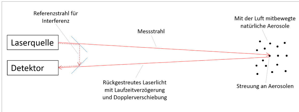
Abb. 1: Messprinzip einer LiDAR-Messung.
