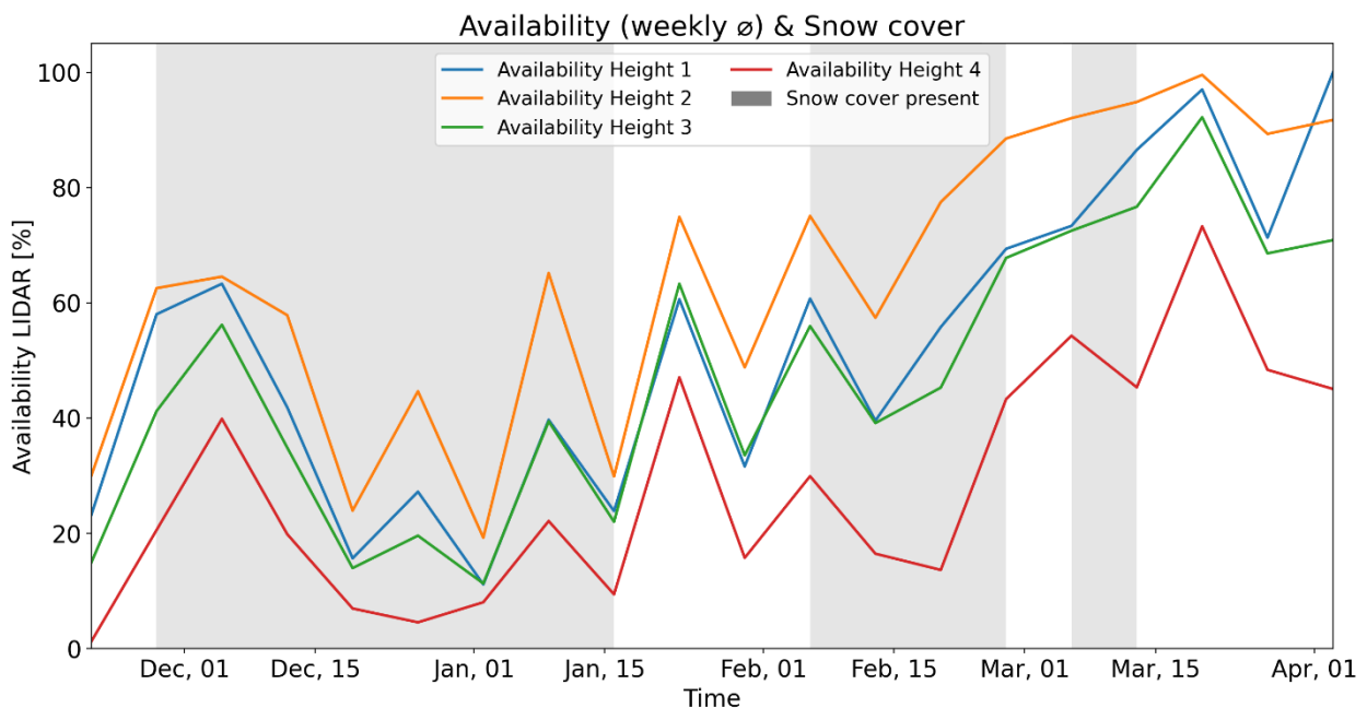
Abb. 3: Beispiel für den Verlauf der wöchentlich durchschnittliche LiDAR-Datenverfügbarkeit und des Vorhandenseins einer Schneedecke an einem Alpinen Standort.
