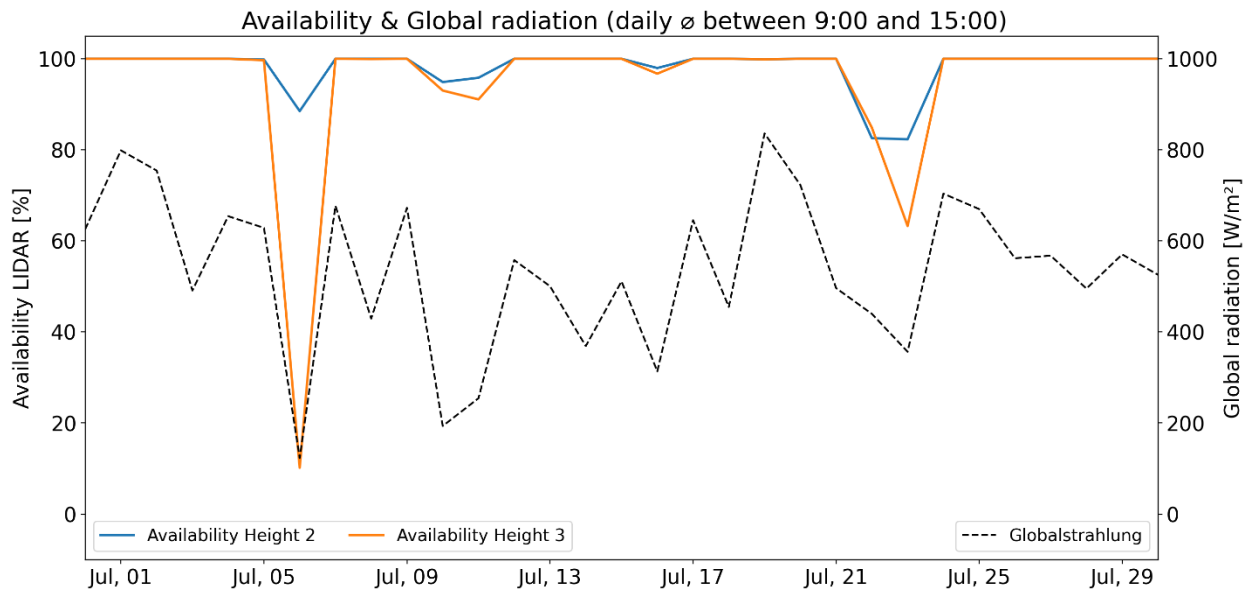
Abb. 9: Gegenüberstellung von LiDAR-Verfügbarkeit und Globalstrahlung im Zeitverlauf für einen Bergstandort.
