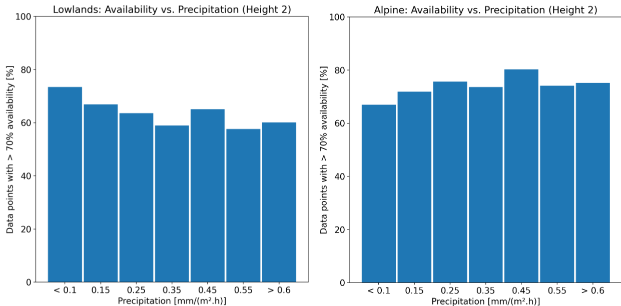
Abb. 5: LIDAR-Verfügbarkeit in Abhängigkeit von der Niederschlagsintensität in Flachlandstandorten (links) und Bergstandorten (rechts).
