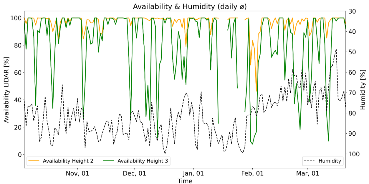
Abb. 6: Beispiel für den Verlauf von LiDAR-Verfügbarkeit und Luftfeuchtigkeit an einem Flachlandstandort.
