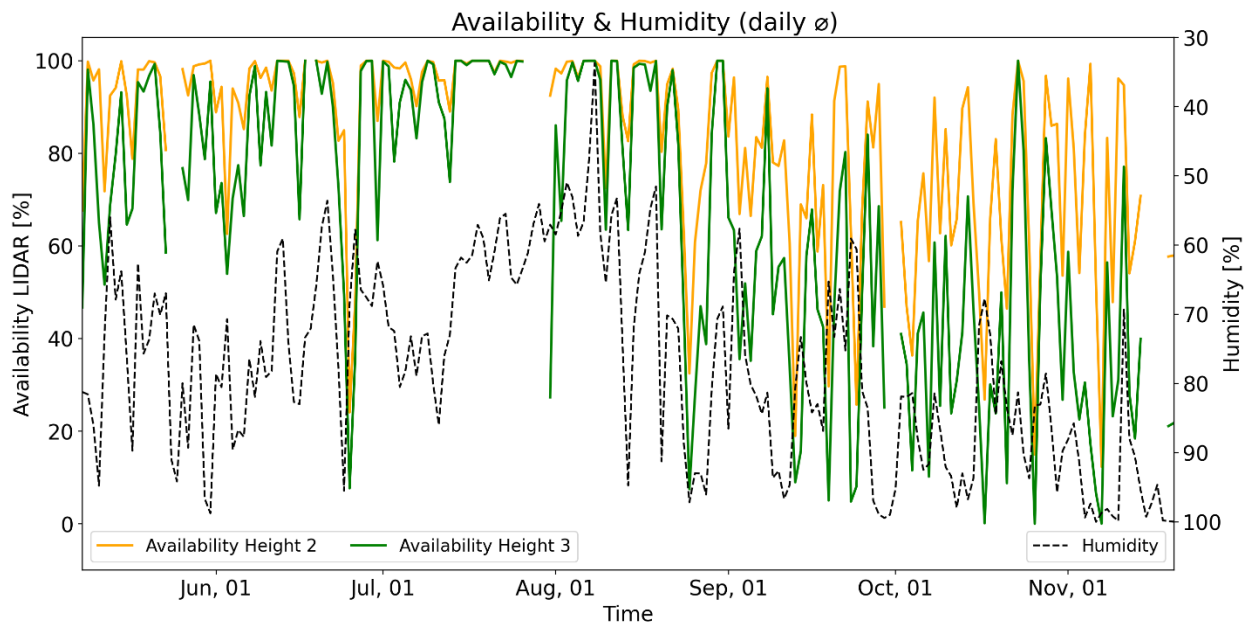
Abb. 7: Beispiel für den Verlauf von LiDAR-Verfügbarkeit und Luftfeuchtigkeit an einem Bergstandort.
