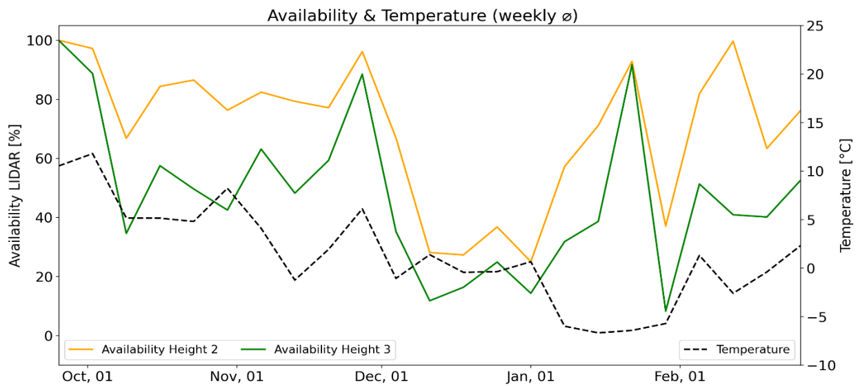
Abb. 11: Beispiel für den Verlauf von Verfügbarkeit und Temperatur an einem Bergstandort.
