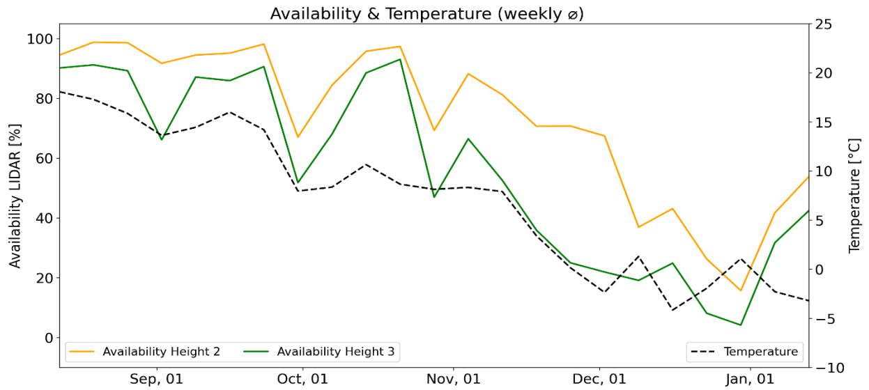
Abb. 10: Beispiel für den Verlauf von Verfügbarkeit und Temperatur an einem Bergstandort.
